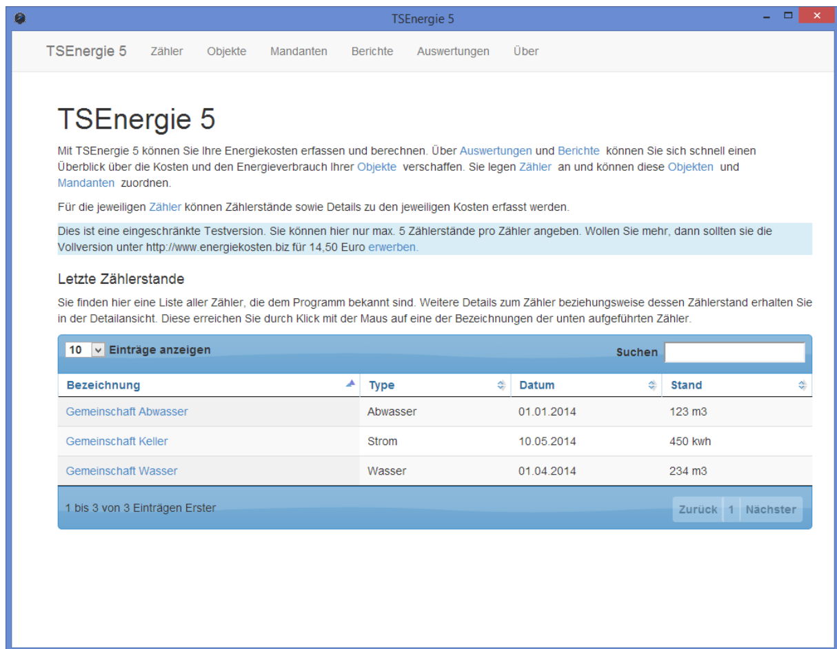
ABBILDUNG 1 HAUPTBILDSCHIRM TSENERGIE 5
